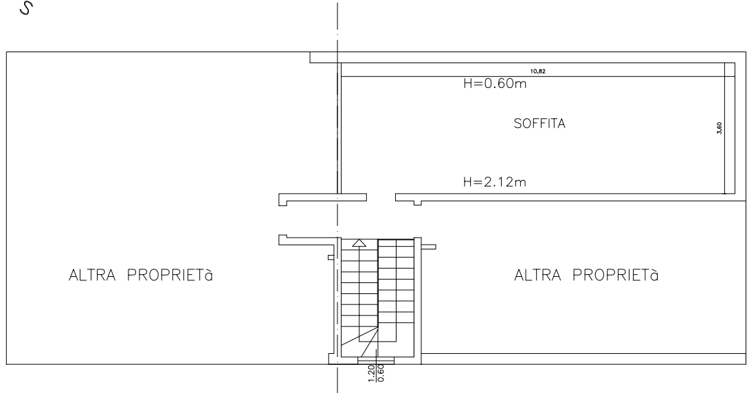
PIANTA PIANO SECONDO - SOFFITA
